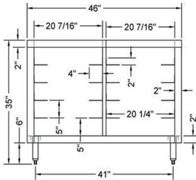
TDR2046 - dimensions
