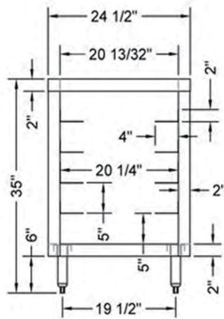
TDR2046 - dimensions
