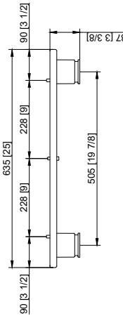
Seitenansicht mit niedrigen Füßen Side view with short feet Vue de côté avec pieds bas
