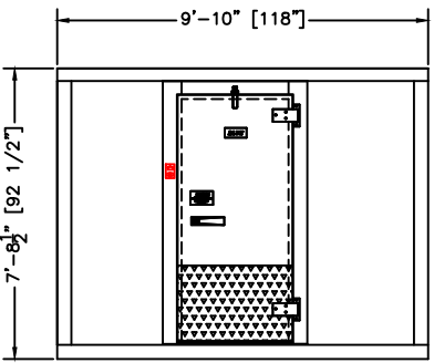
ELEVATION RIGHT HINGE
