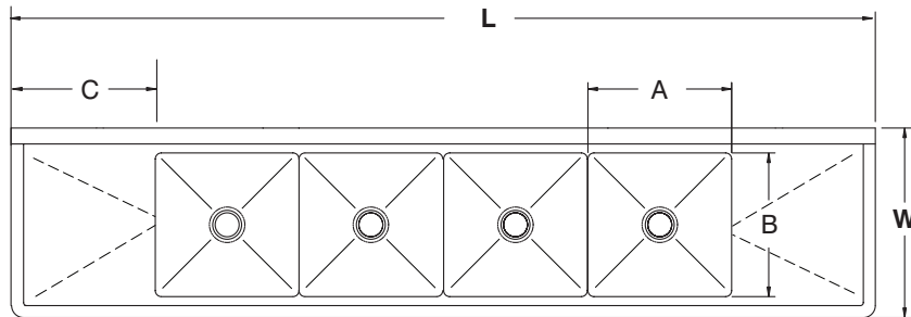
4 COMP - 2 DRBD
