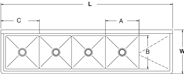
4 COMP - 1 DRBD
