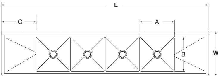
4 COMP - 2 DRBDS
