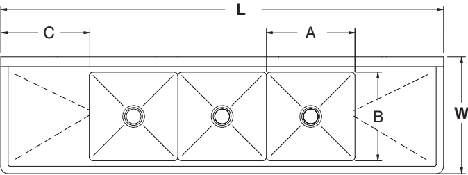
3 COMP - 2 DRBD
