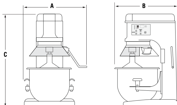
7/10 Quart Mixer
