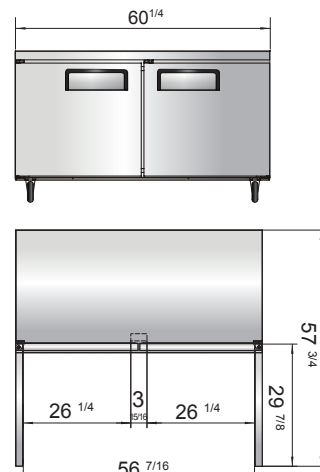
MGF8407GR
