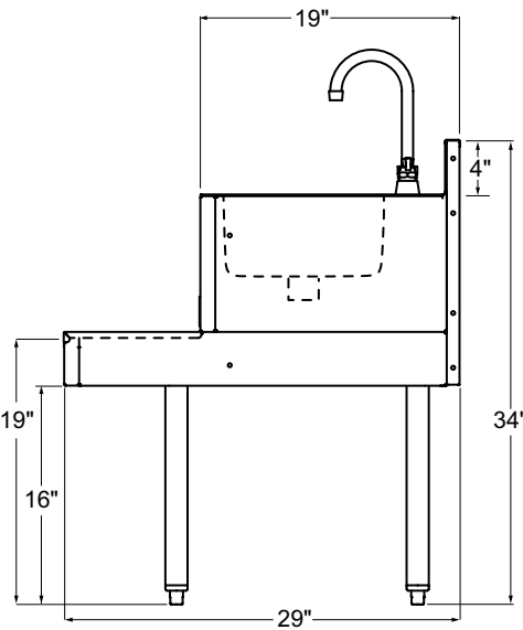
C-BSB-12, C-BSB-14, C-BSB-18 SIDE ELEVATION
