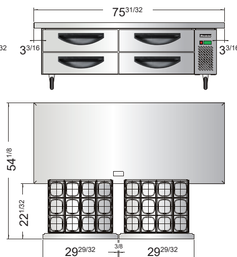
PDRB-76T-HC
