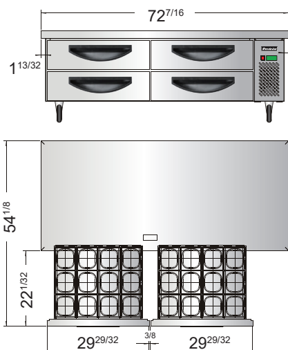
PDRB-72-HC
