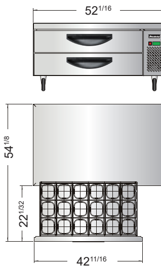
PDRB-76T-HC
