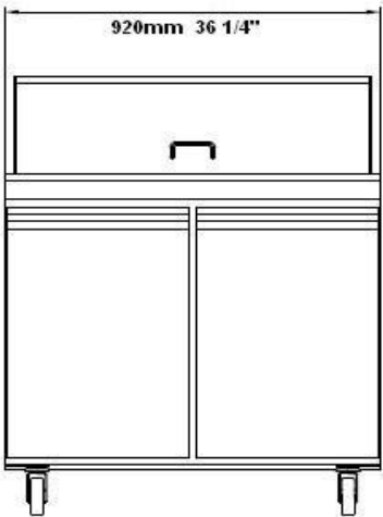
Elevation
