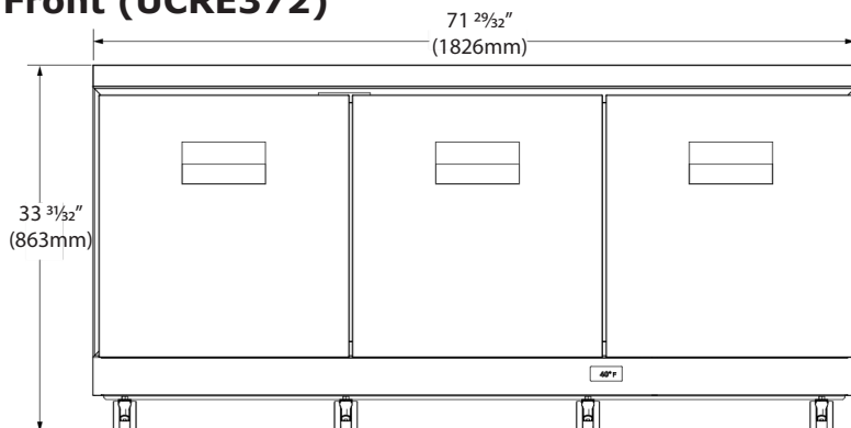
Front (UCRE372)
