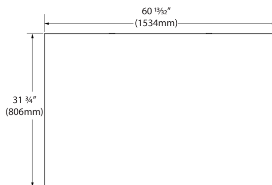
Top (UCRE360)
